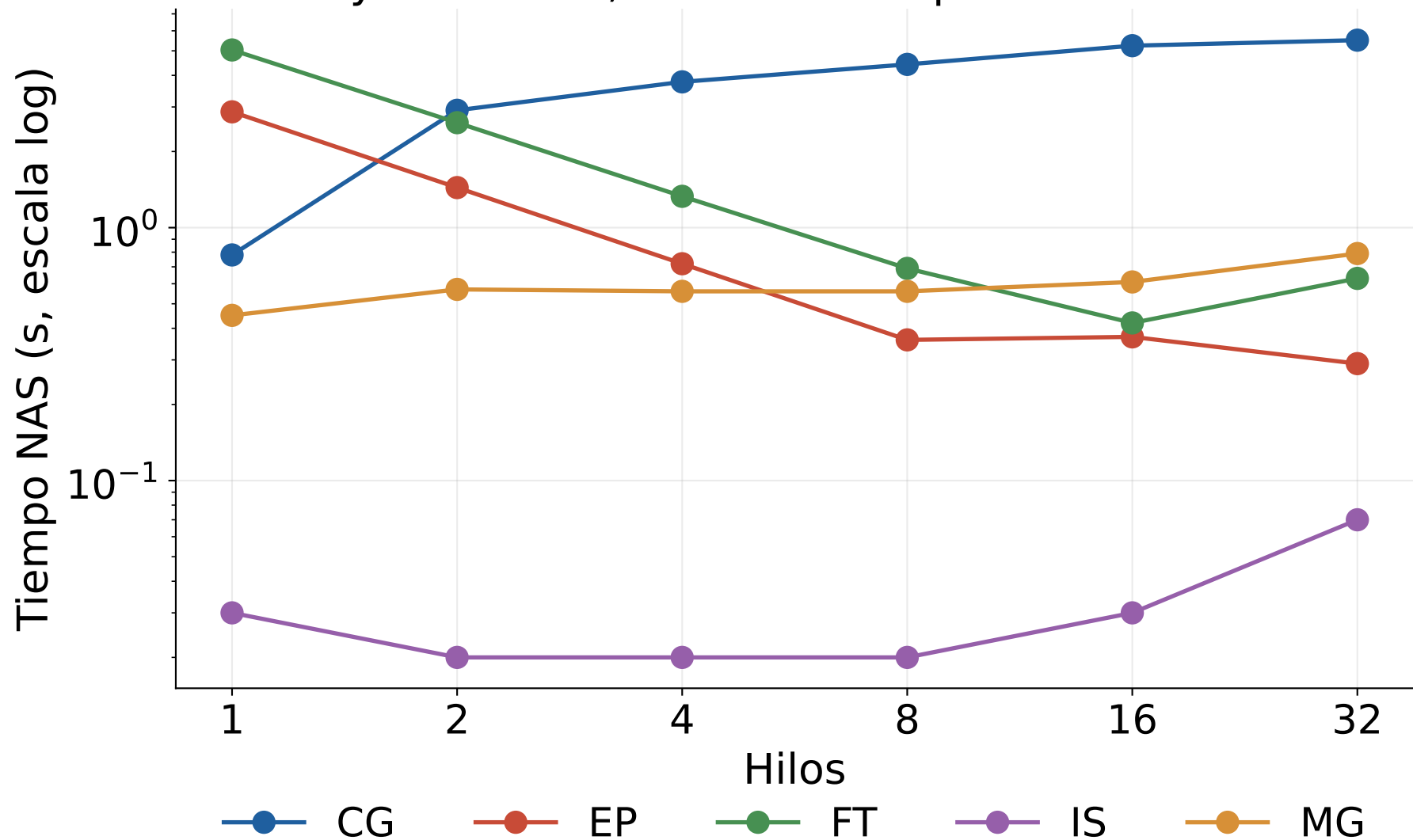
Python 3.15t, modo 3: tiempos en clase W
