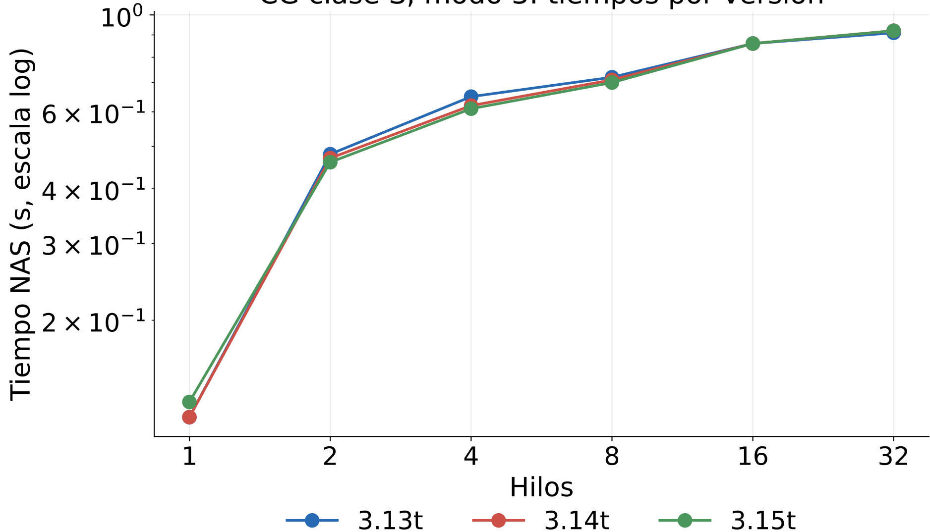
CG clase S, modo 3: tiempos por versión
