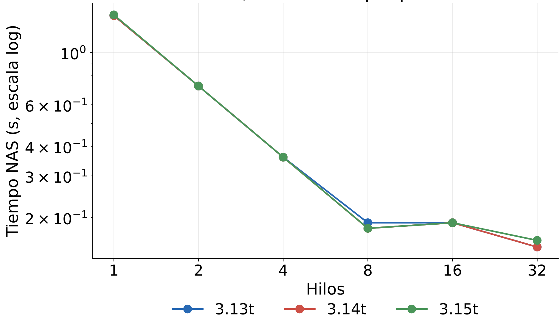
EP clase S, modo 3: tiempos por versión
