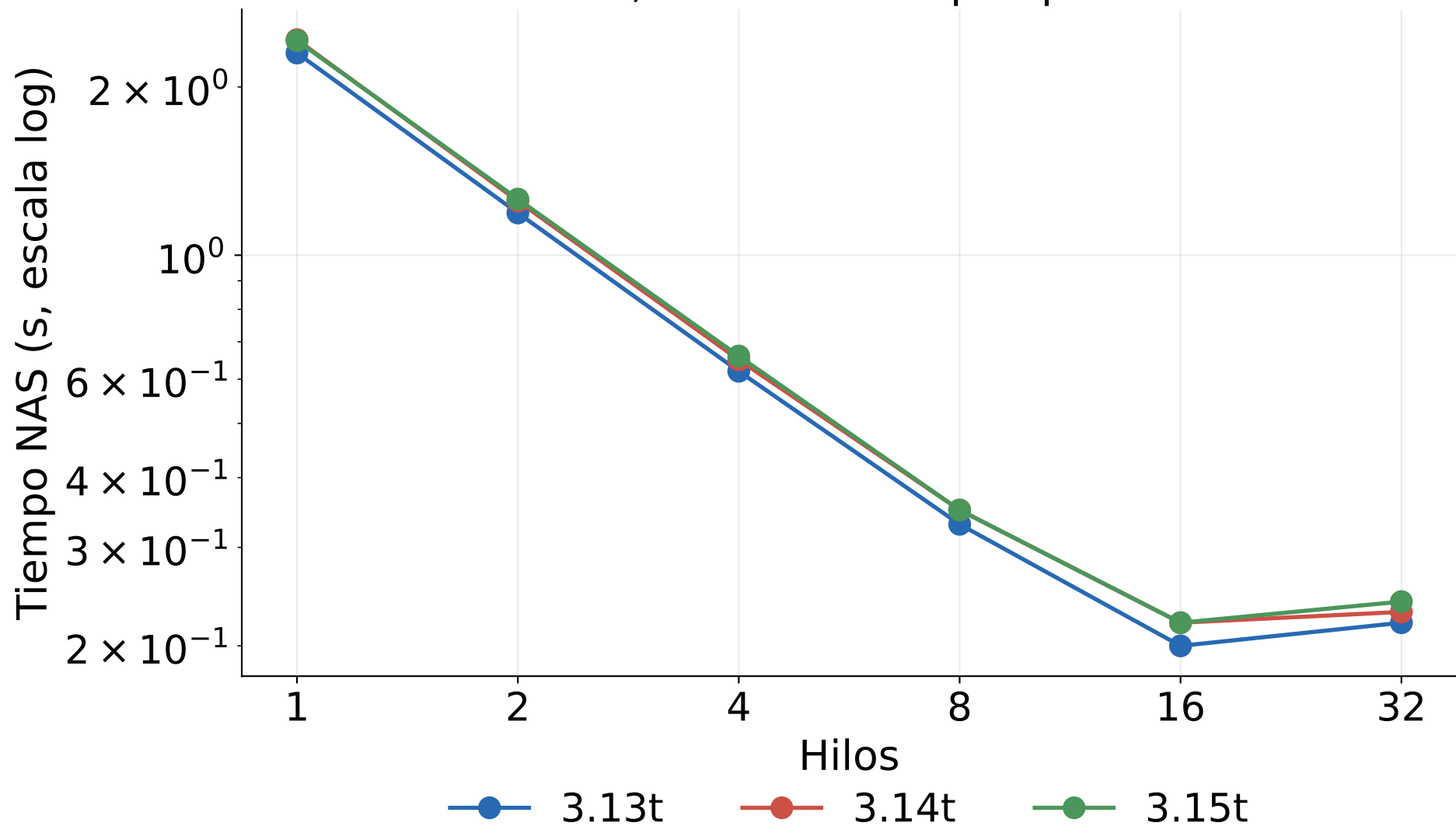
FT clase S, modo 3: tiempos por versión
