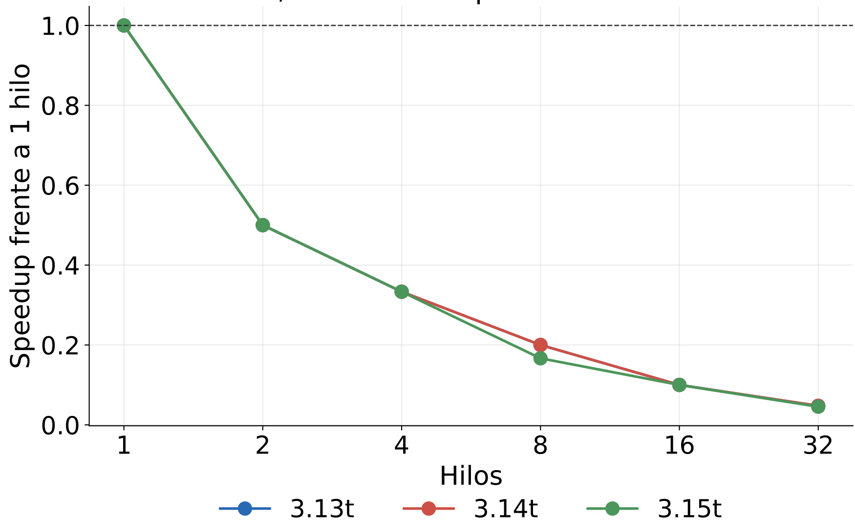
MG clase S, modo 3: comparación entre versiones
