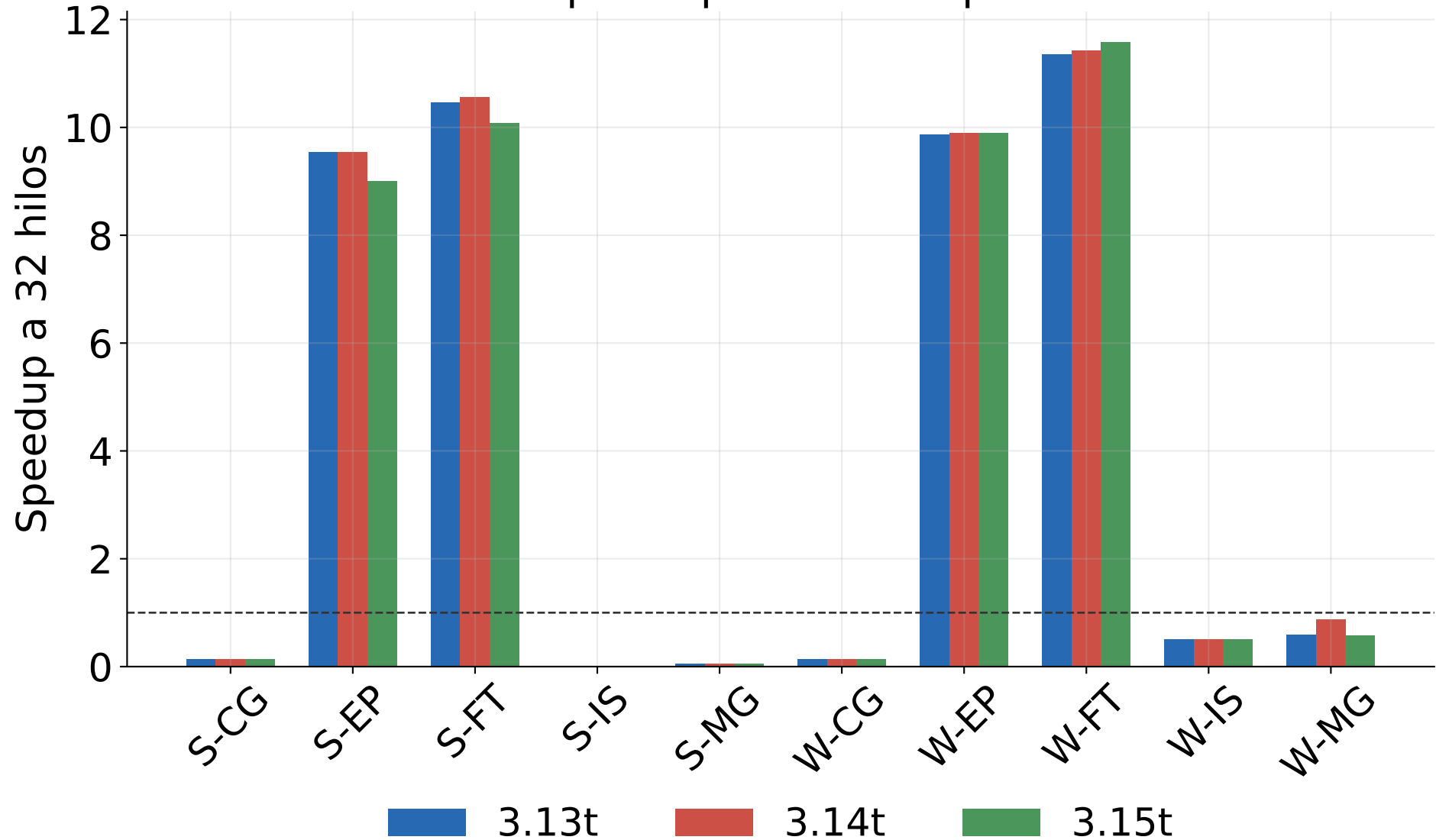
Modo 3: speedup a 32 hilos por versión
