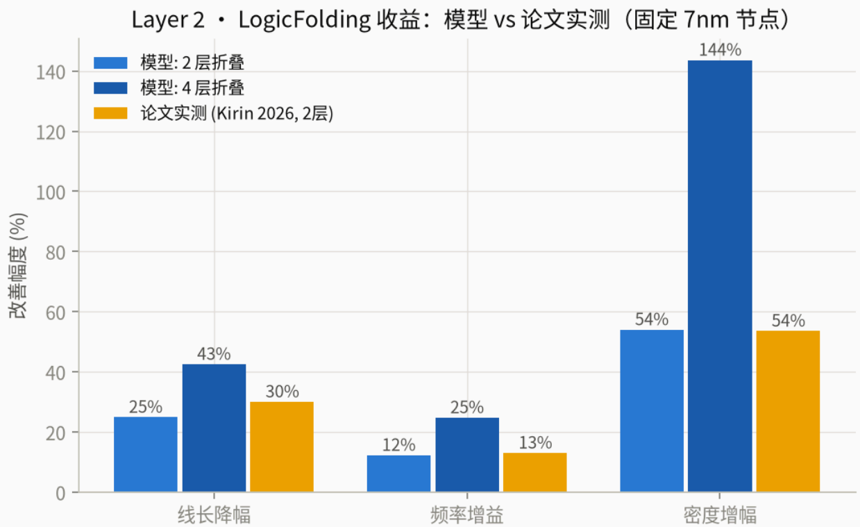
图 3 · 电路层: LogicFolding 收益，模型（独立文献参数） vs Kirin 2026 实测
