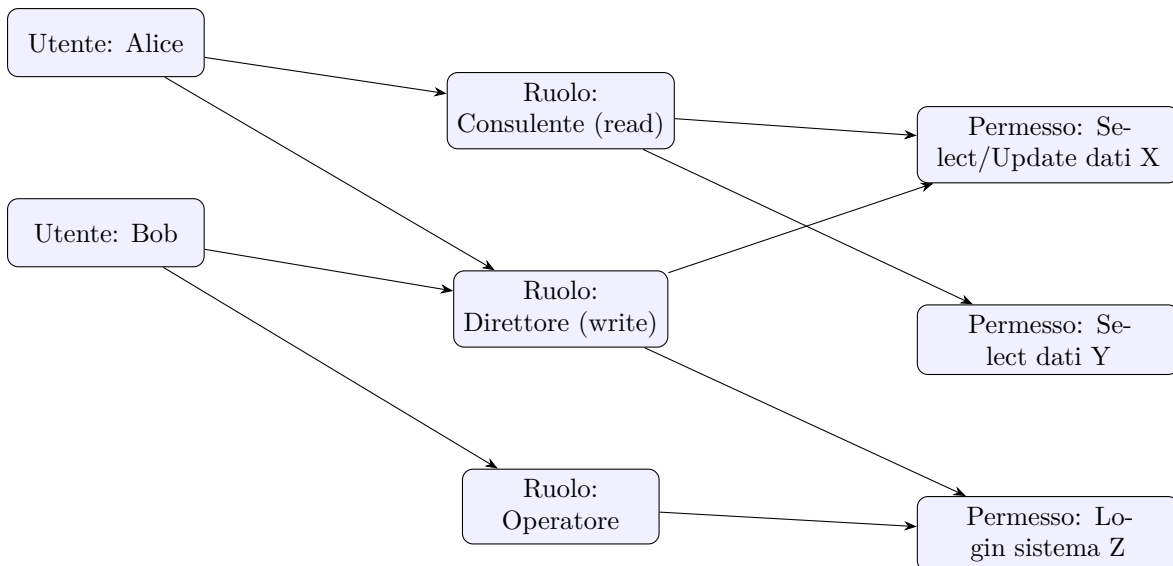
Figura 4: RBAC: relazione molti-a-molti tra utenti, ruoli e permessi – il ruolo è il livello di astrazione intermedio che disaccoppia utenti e permessi.
