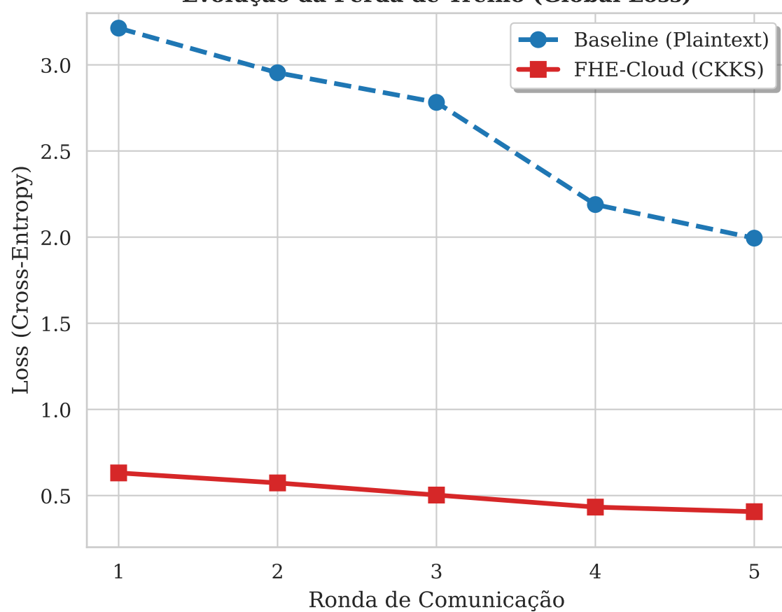
Evolução da Perda de Treino (Global Loss)
