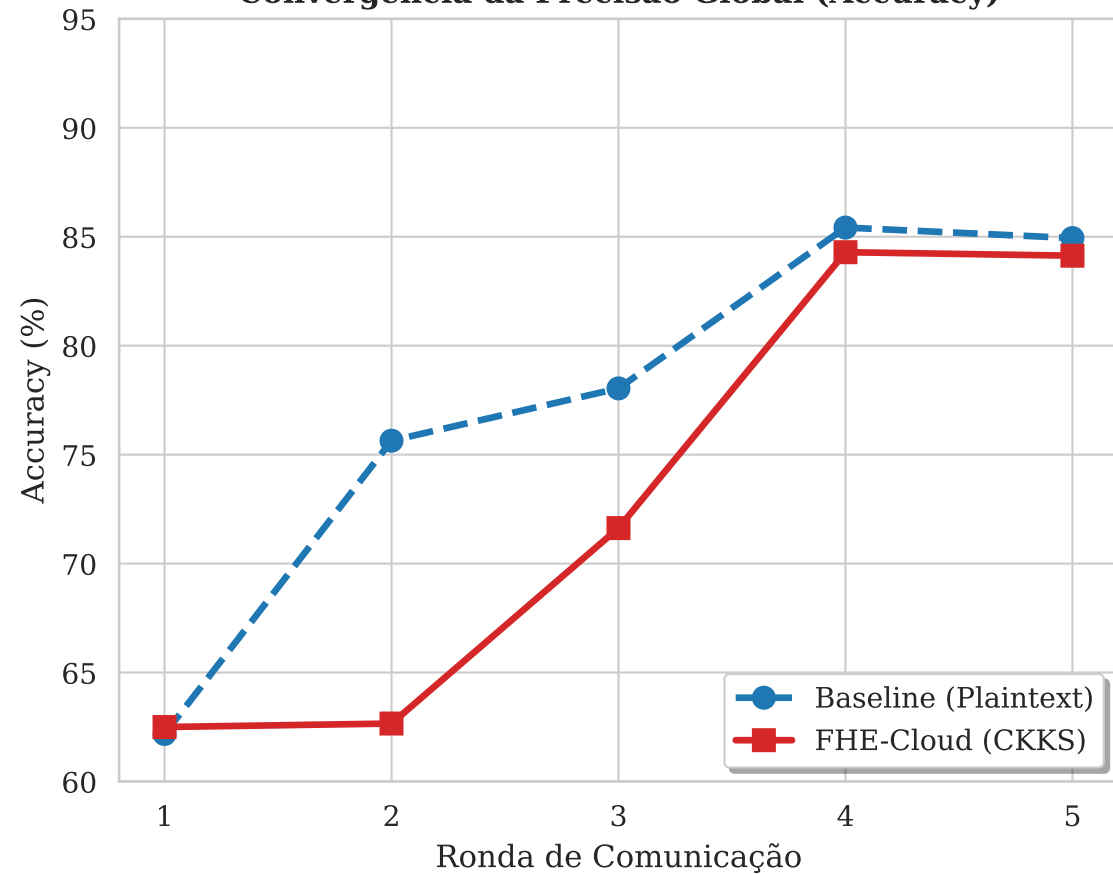
Convergência da Precisão Global (Accuracy)
