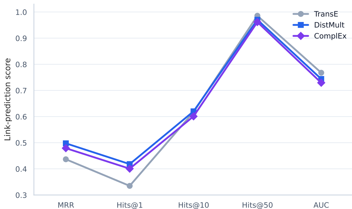
YAGO
