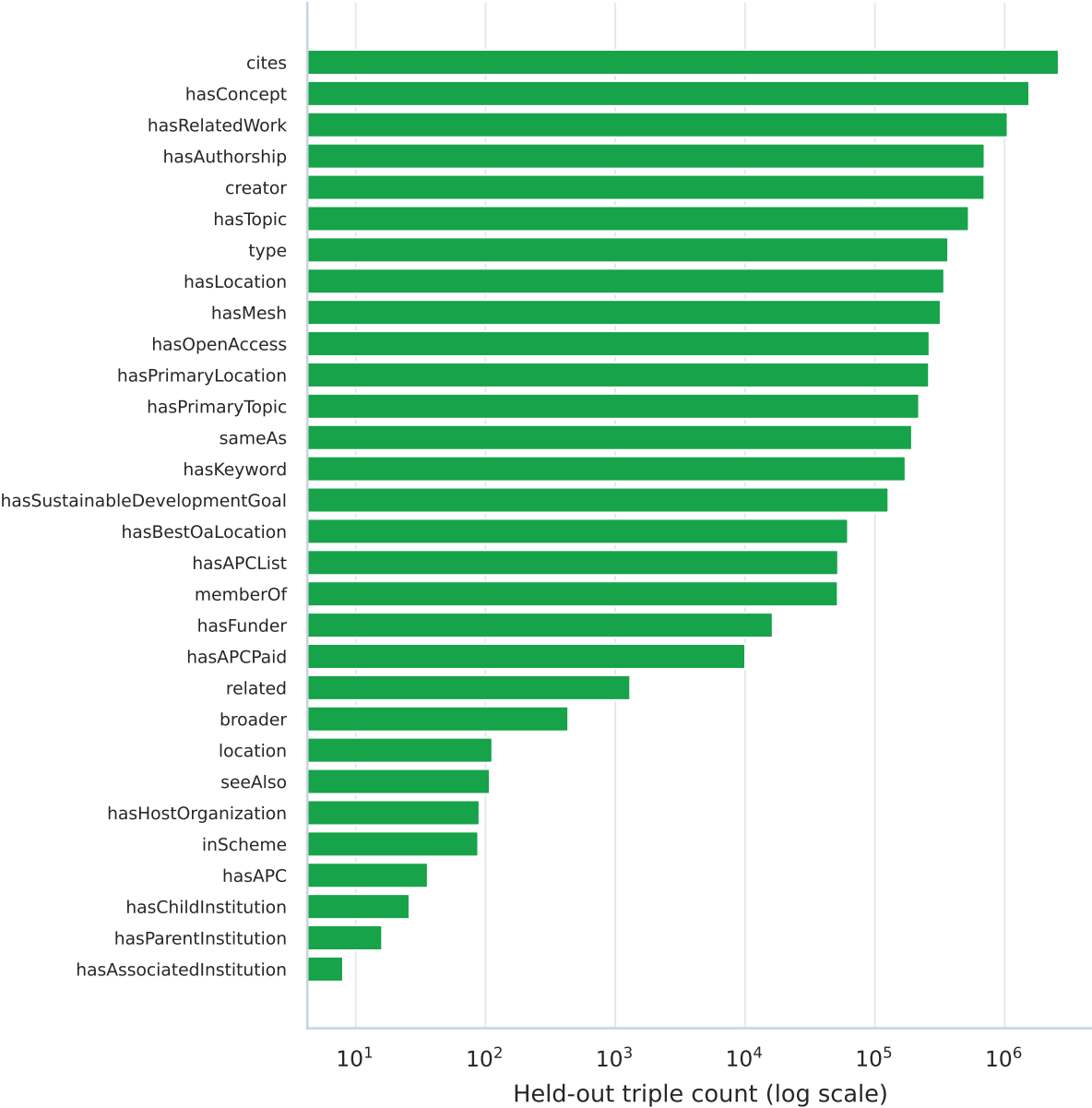
SemOpenAlex
