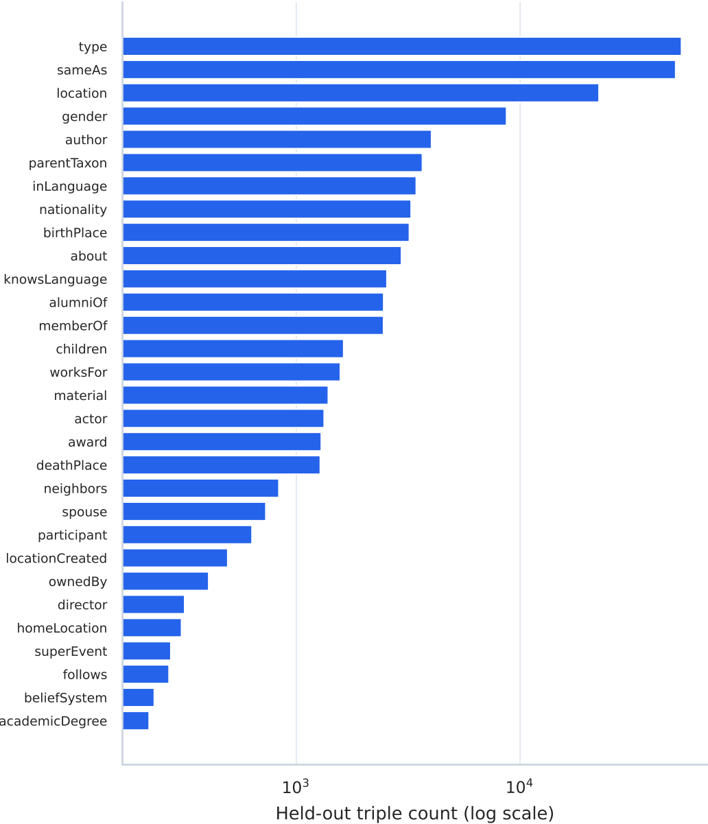
YAGO
