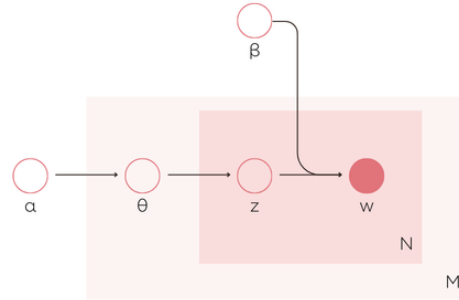
Figura 11: Representación gráfica de LDA
