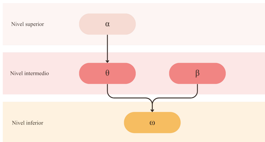
Figura 3: Diagrama del flujo de un modelo jer3rquico a 3 niveles con dos grupos
