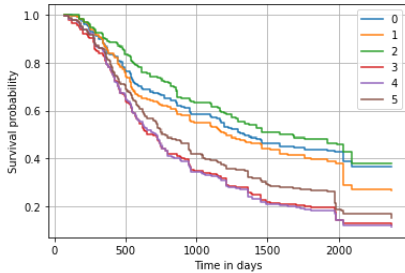
Figura 3: Ejemplo de curvas de supervivencia predichas mediante Random Survival Forest. Fuente: documentación oficial de scikit-survival [15].
