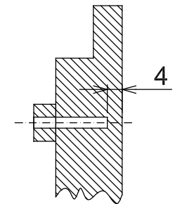
B-B' SCALE : 2 : 1
