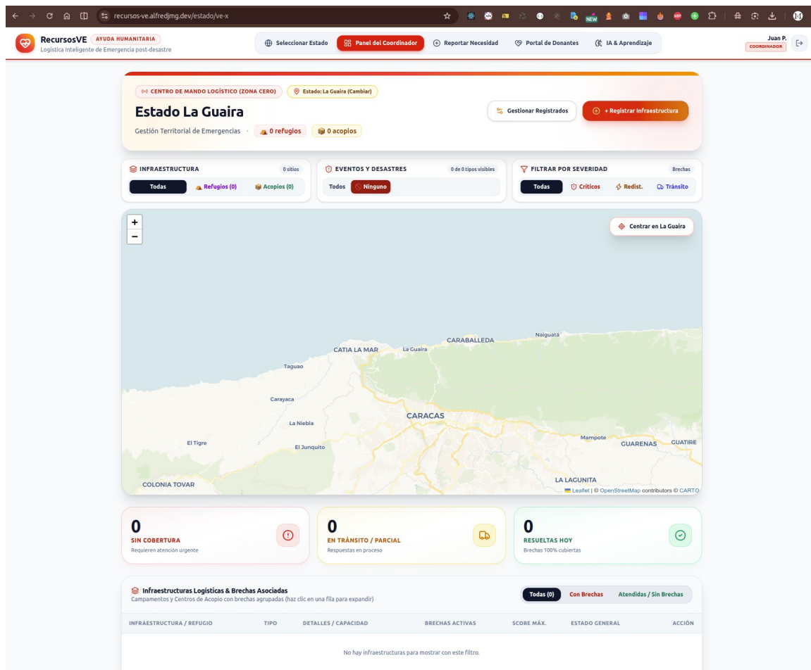
Figura 3. Dashboard Principal del Centro de Mando Logístico con Mapa Real Leaflet y Zonas de Impacto
