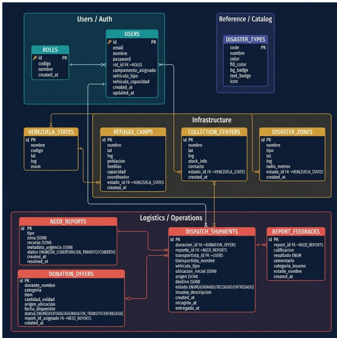
Figura 3b. Diagrama de Entidad-Relación (ER) — Base de Datos PostgreSQL de RecursosVE
