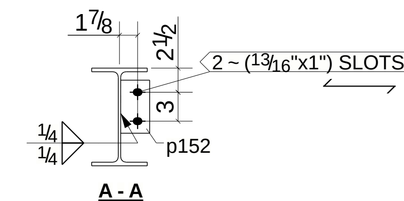
2 - BEAMS - 614B2
