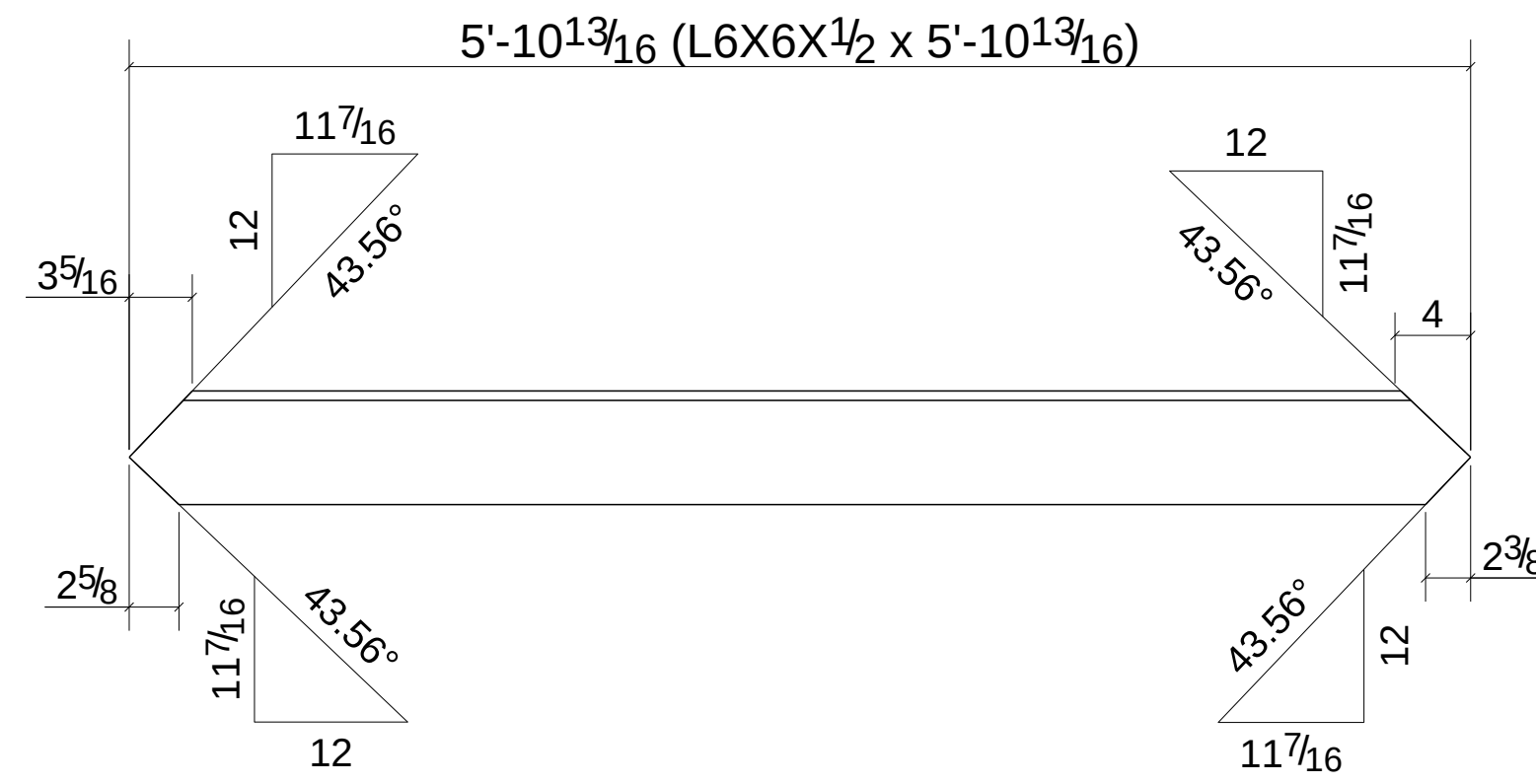
2 - HORIZONTAL BRACES - 640HB2
