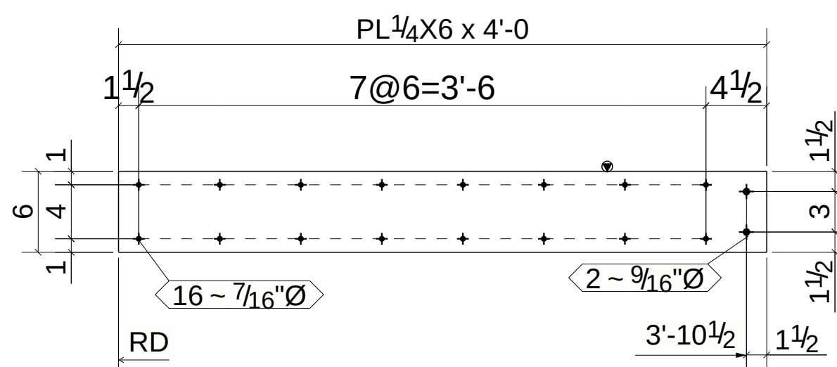
2 - DRAG PLATES - 645PL5
