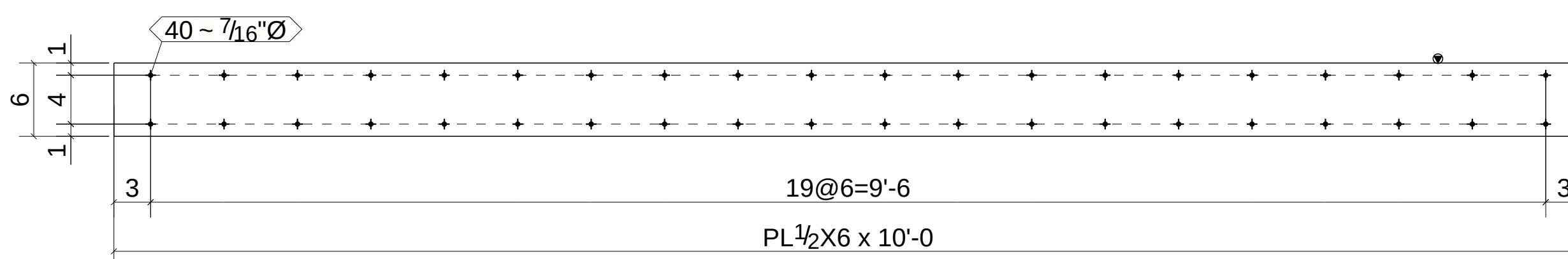
4 - DRAG PLATES - 645PL3
