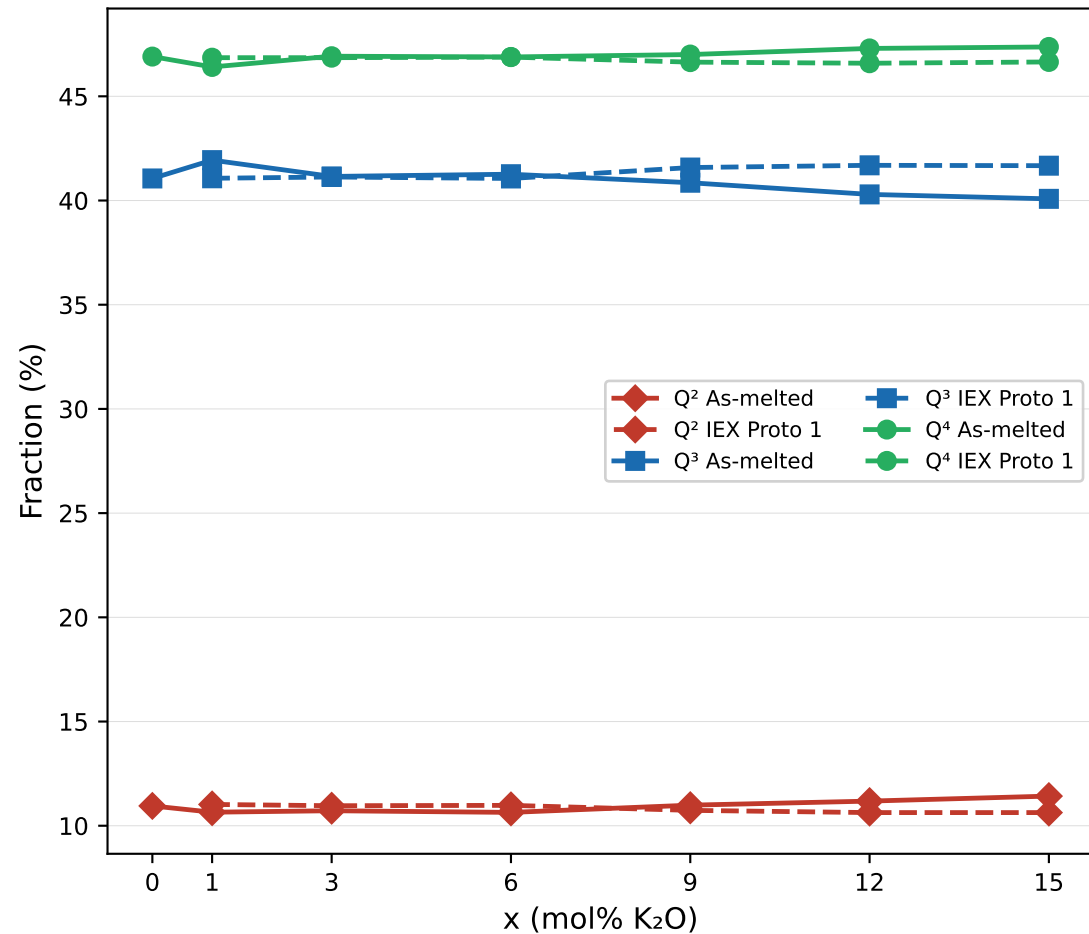
As-melted vs IEX Proto1
