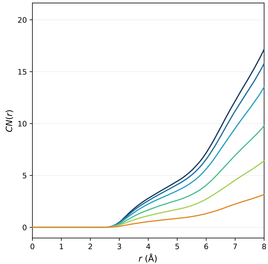
CN(r) — Ca-Na
