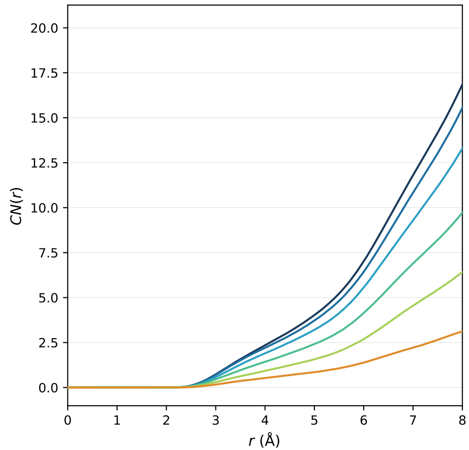
CN(r) — Na-Na
