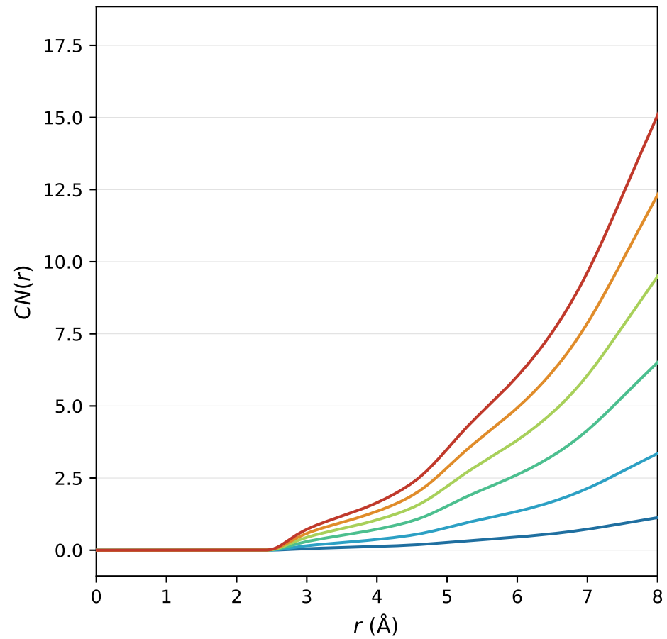
CN(r) — O-K
