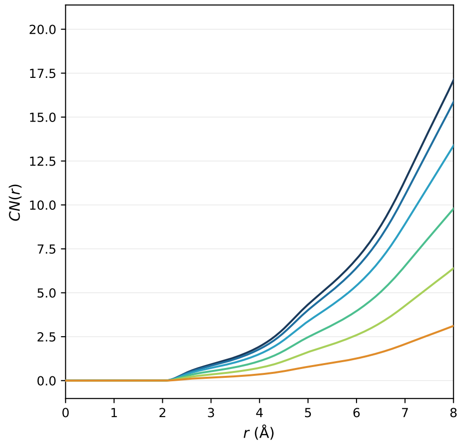
CN(r) — O-Na
