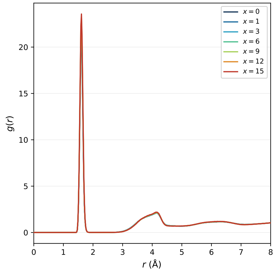
g(r) — Si-O
