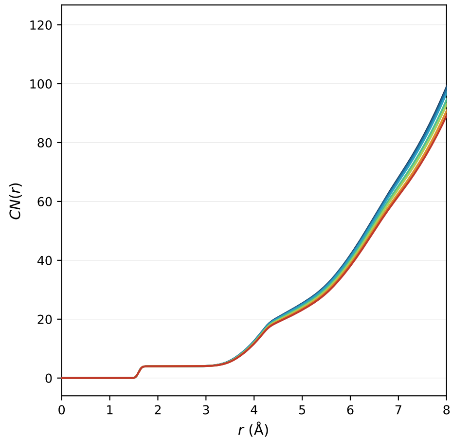
CN(r) — Si-O
