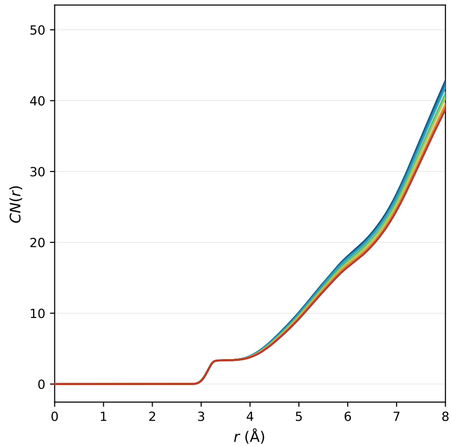
CN(r) — Si-Si
