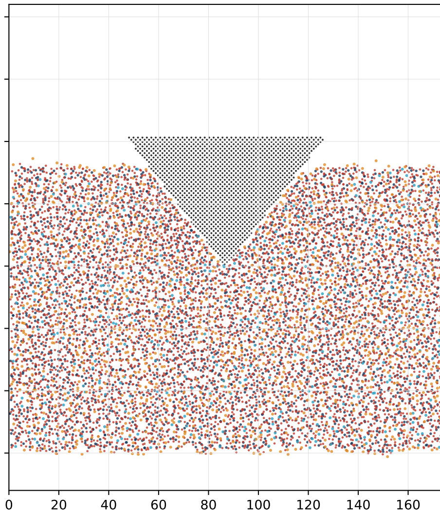
Corte transversal ( |y-y_{\text{mid}}| < 3.5 \text{ \AA} ) — CaO x=0 r=1 , geometría corregida (DEVANA)
