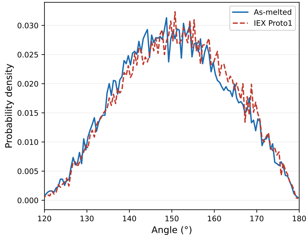
Si-O-Si
