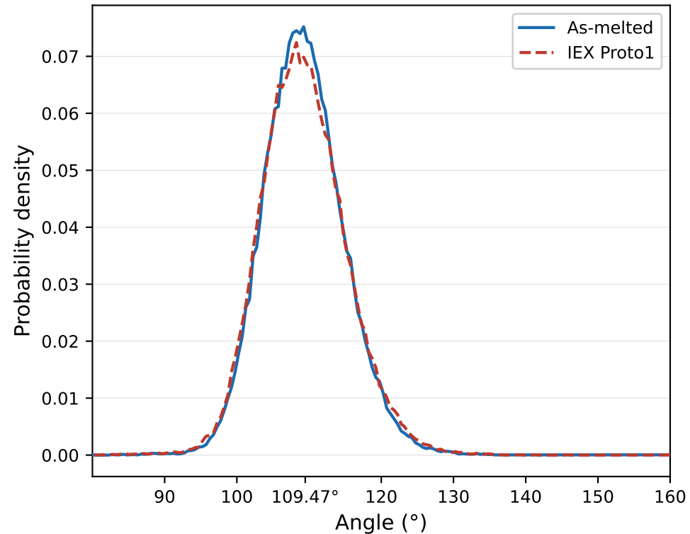
O-Si-O
