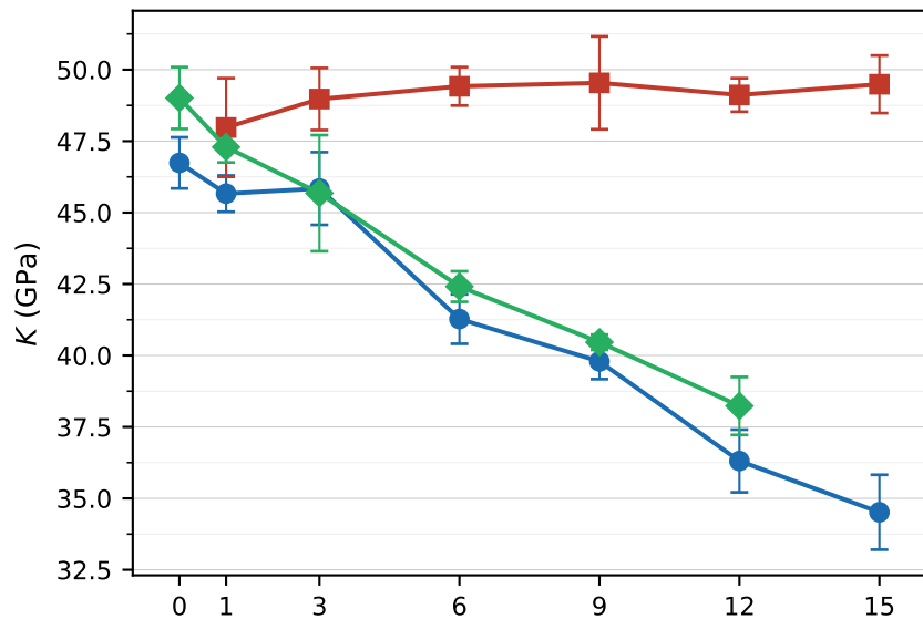
PMMC r_c = 8 \text{ \AA} — Propiedades elásticas adiabáticas ( T = 0 \text{ K} | 300 \text{ K} ) 75\text{SiO}_2 \cdot (15-x)\text{Na}_2\text{O} \cdot x\text{K}_2\text{O} \cdot 10\text{CaO}
