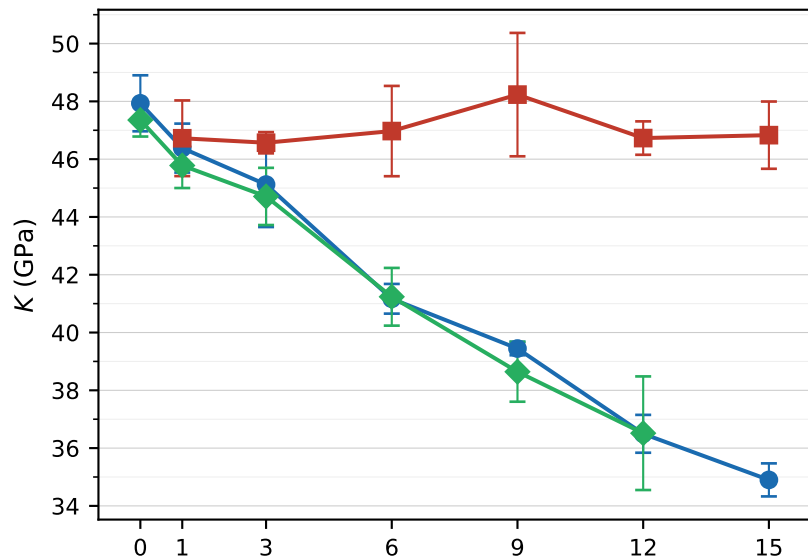
PMMCS r_c = 8 \text{ \AA} — Propiedades elásticas adiabáticas ( T = 0 \text{ K} ) | 723 \text{ K} 75\text{SiO}_2 \cdot (15-x)\text{Na}_2\text{O} \cdot x\text{K}_2\text{O} \cdot 10\text{CaO}
