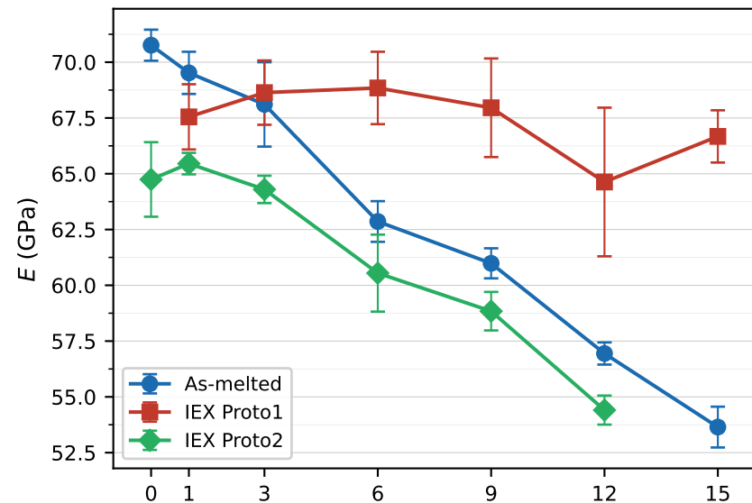
PMMCS r_c = 8 \text{ \AA} — Propiedades elásticas adiabáticas ( T = 0 \text{ K} ) | 723 \text{ K} 75\text{SiO}_2 \cdot (15-x)\text{Na}_2\text{O} \cdot x\text{K}_2\text{O} \cdot 10\text{CaO}
