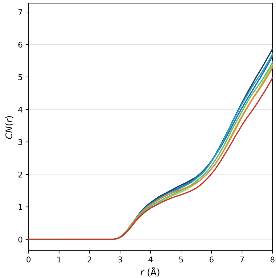
CN(r) — Ca-Ca
