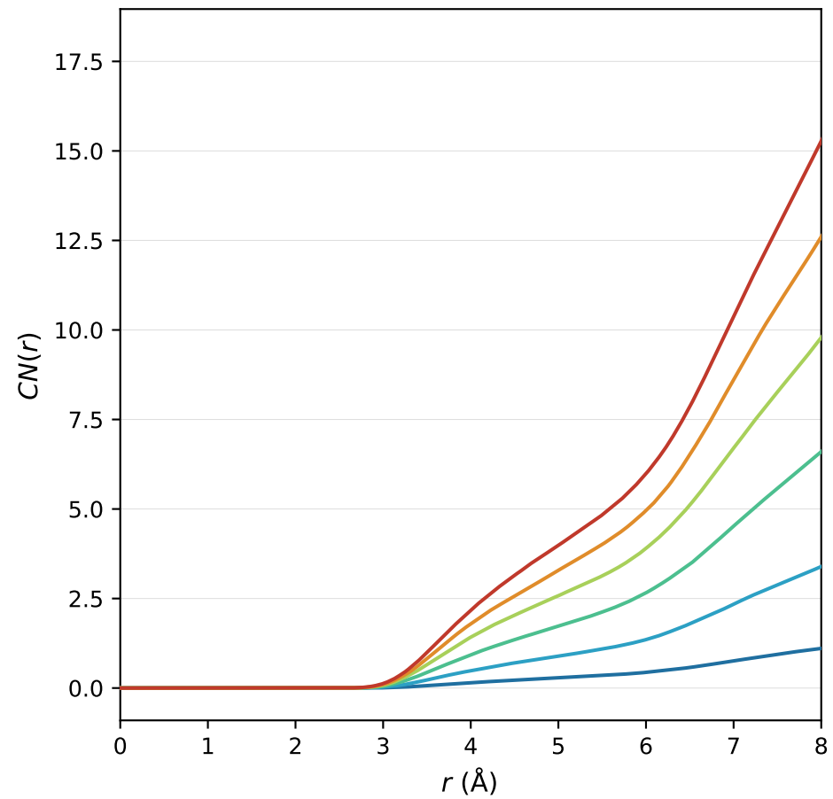
CN(r) — Ca-K
