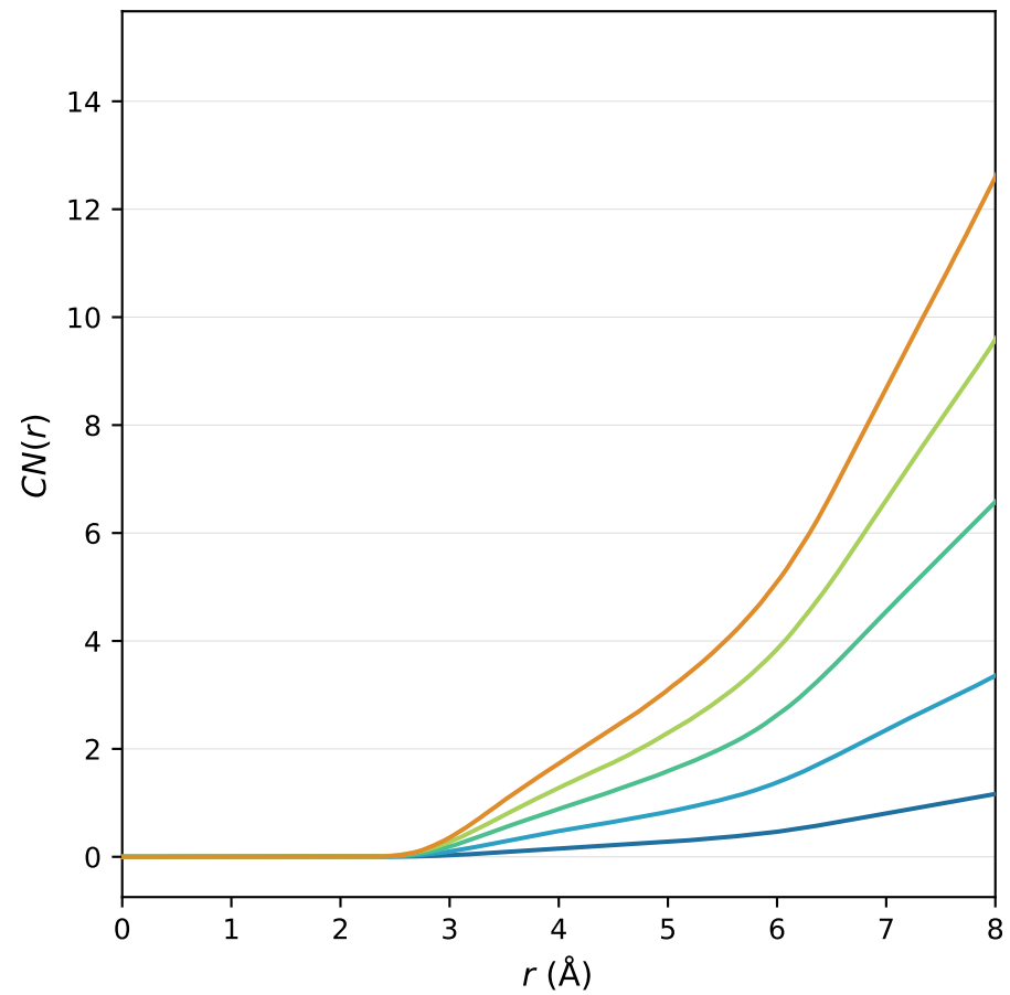
CN(r) — Na-K
