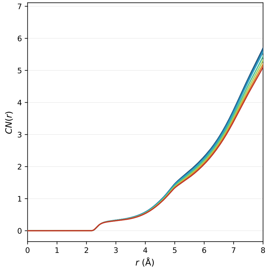
CN(r) — O-Ca
