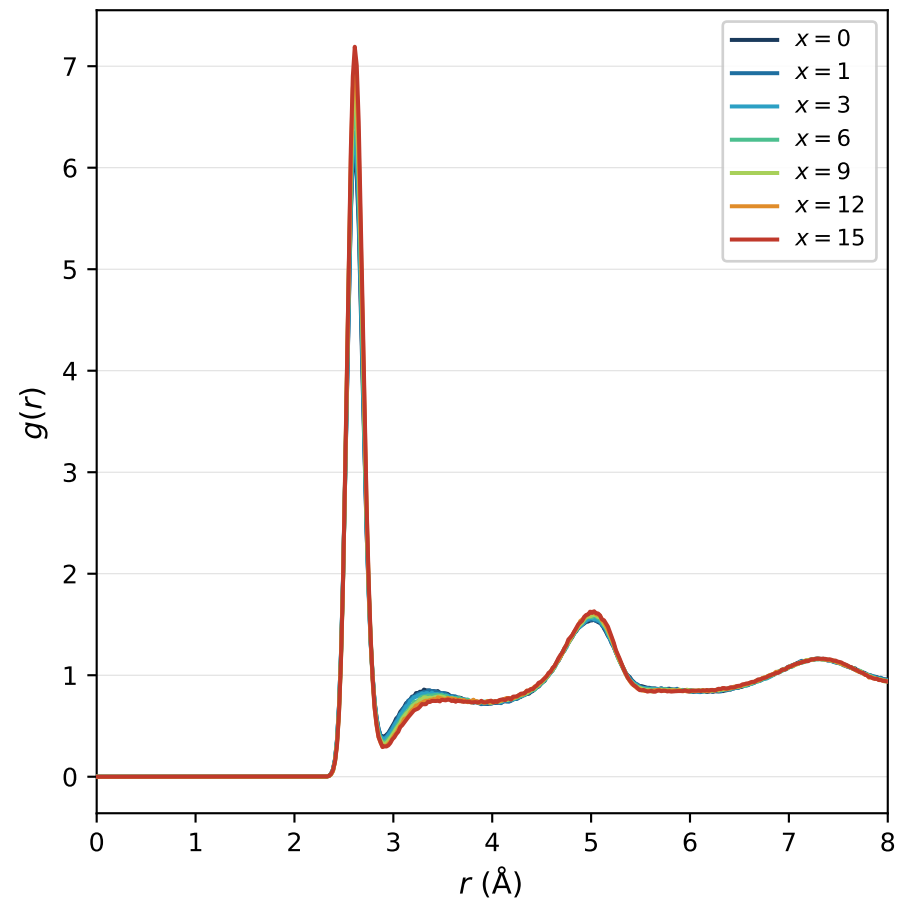
g(r) — O-O
