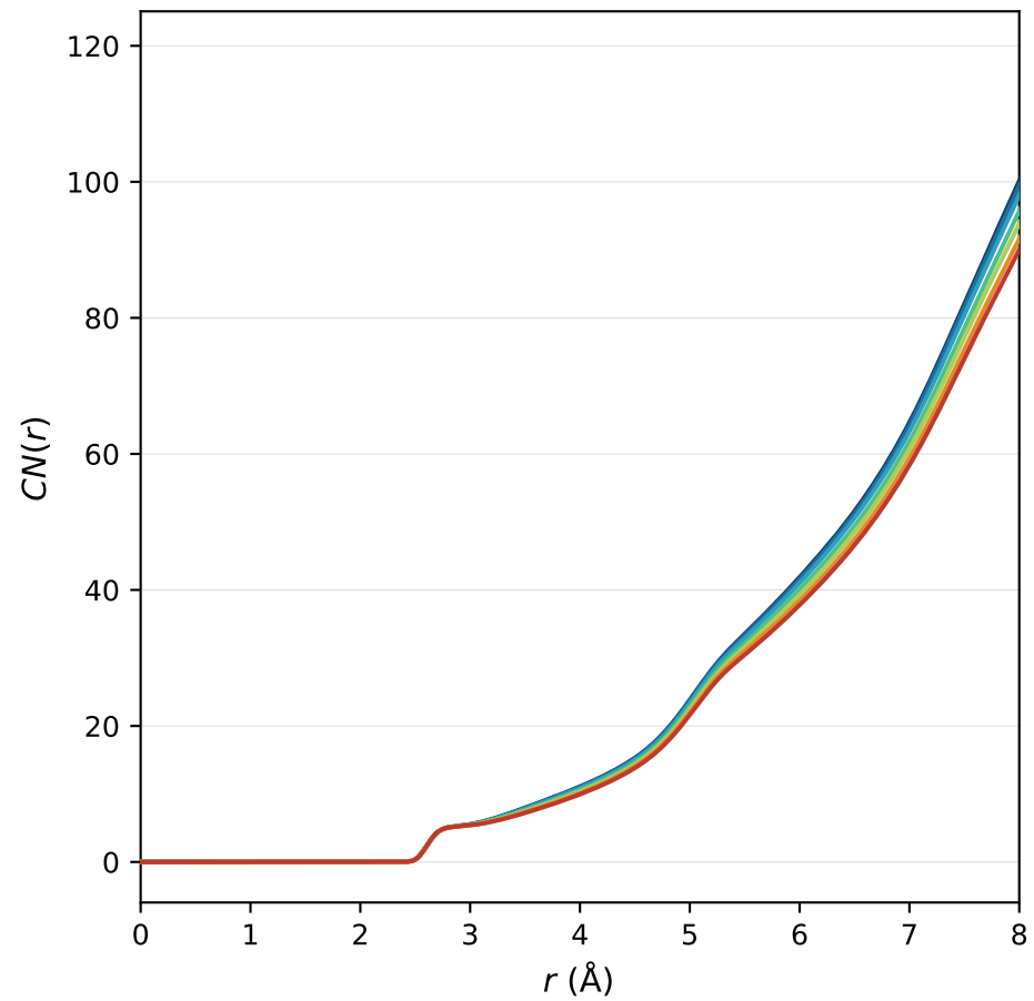
CN(r) — O-O
