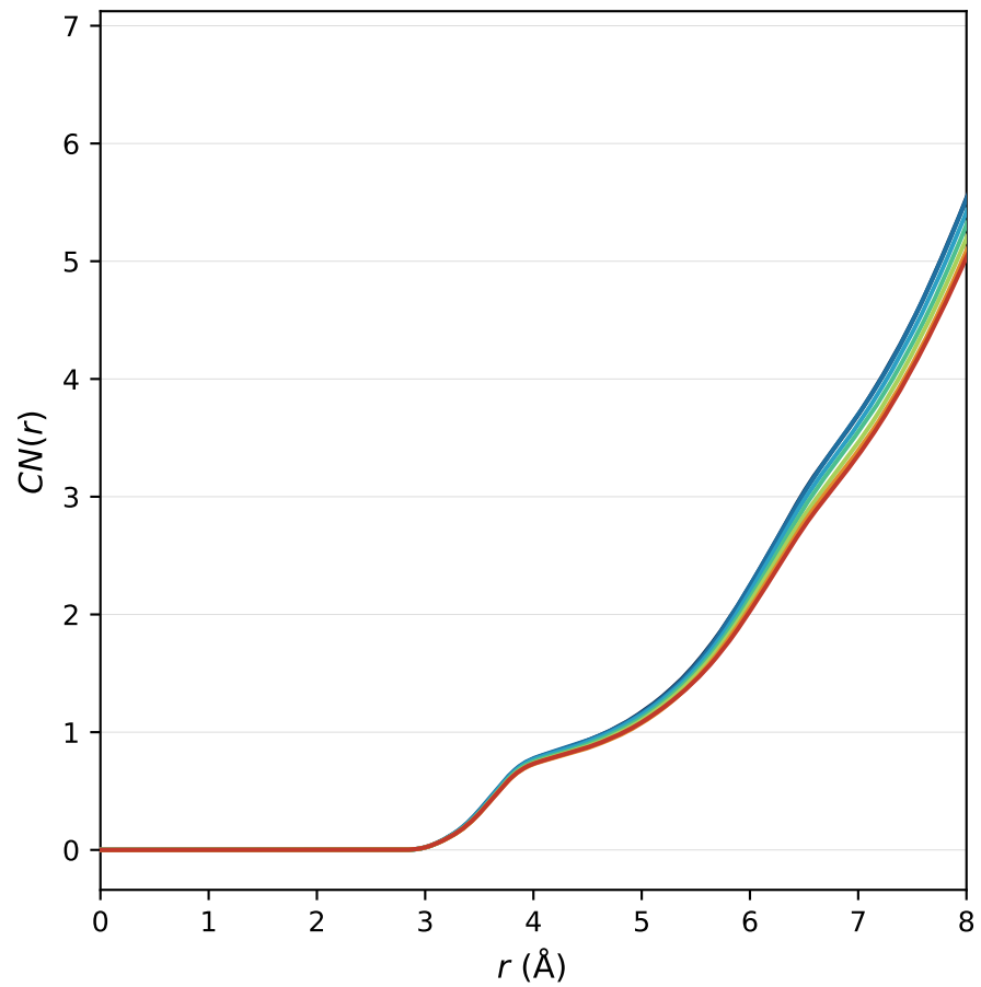
CN(r) — Si-Ca
