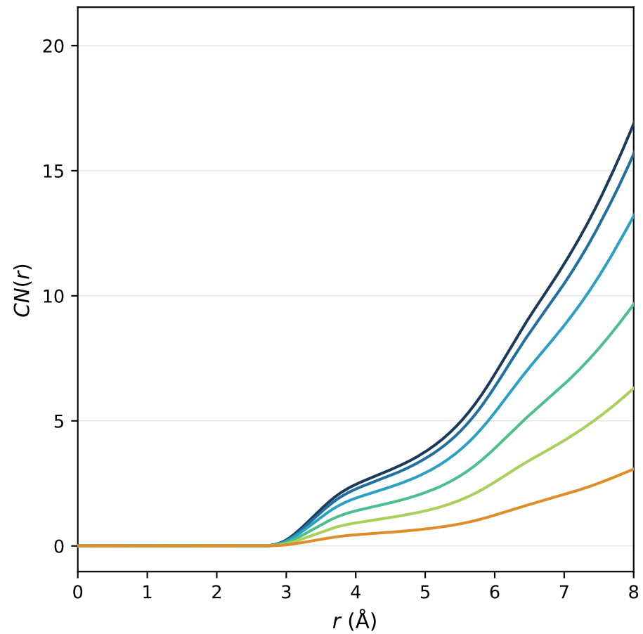
CN(r) — Si-Na
