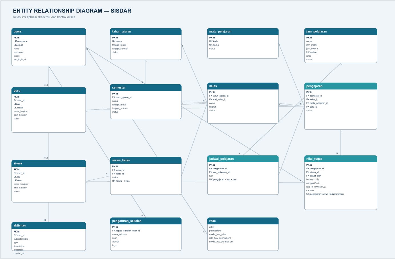
Gambar 1. ERD inti SISDAR. Notasi 1 menunjukkan satu record dan N menunjukkan banyak record.
