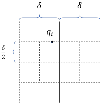
图 8.1: 最近点对问题
