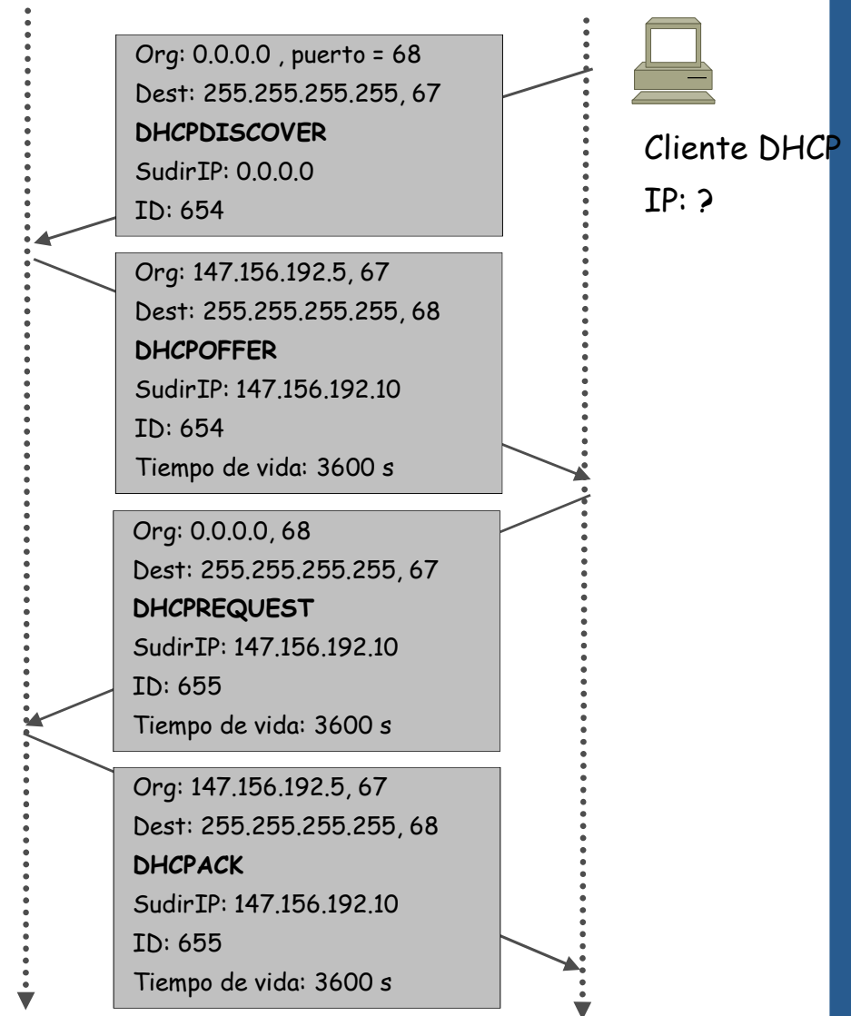
Servidor DHCP 147.156.192.5
