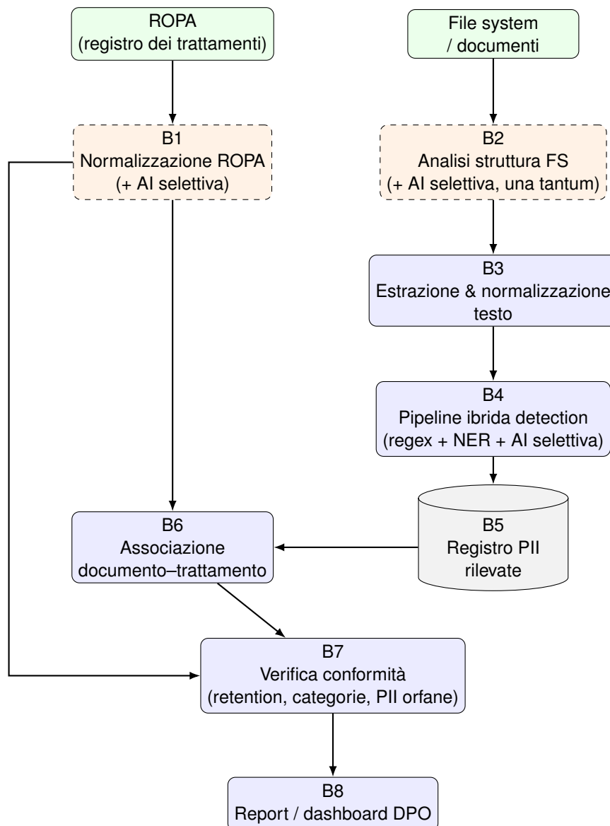
Figura 6.1: Architettura a macro-blocchi del sistema
