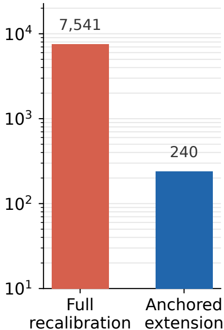
Trainable parameters
