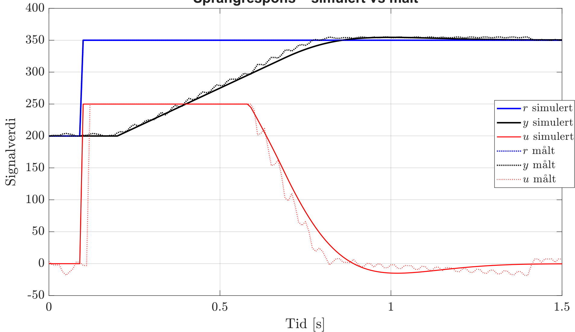
Sprangrespons – simulert vs målt
