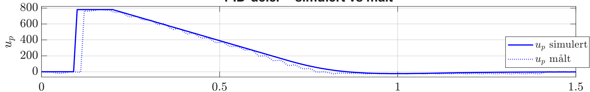
PID-deler – simulert vs målt
