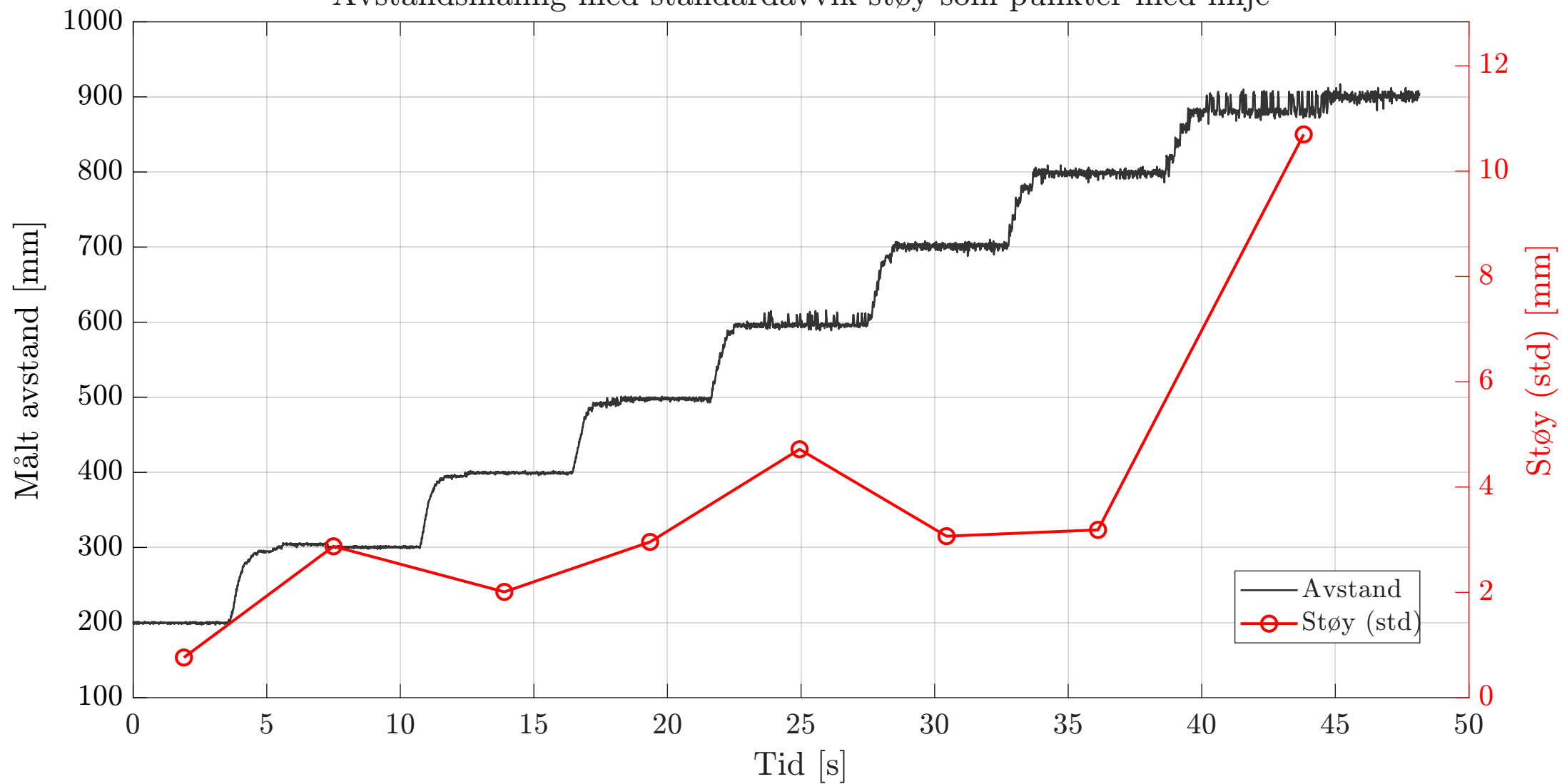
Avstandsmåling med standardavvik støy som punkter med linje
