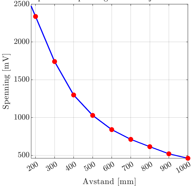
Lookup-tabell: Spenning som funksjon av avstand
