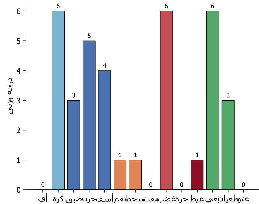
الف) مرکزیت درجه
