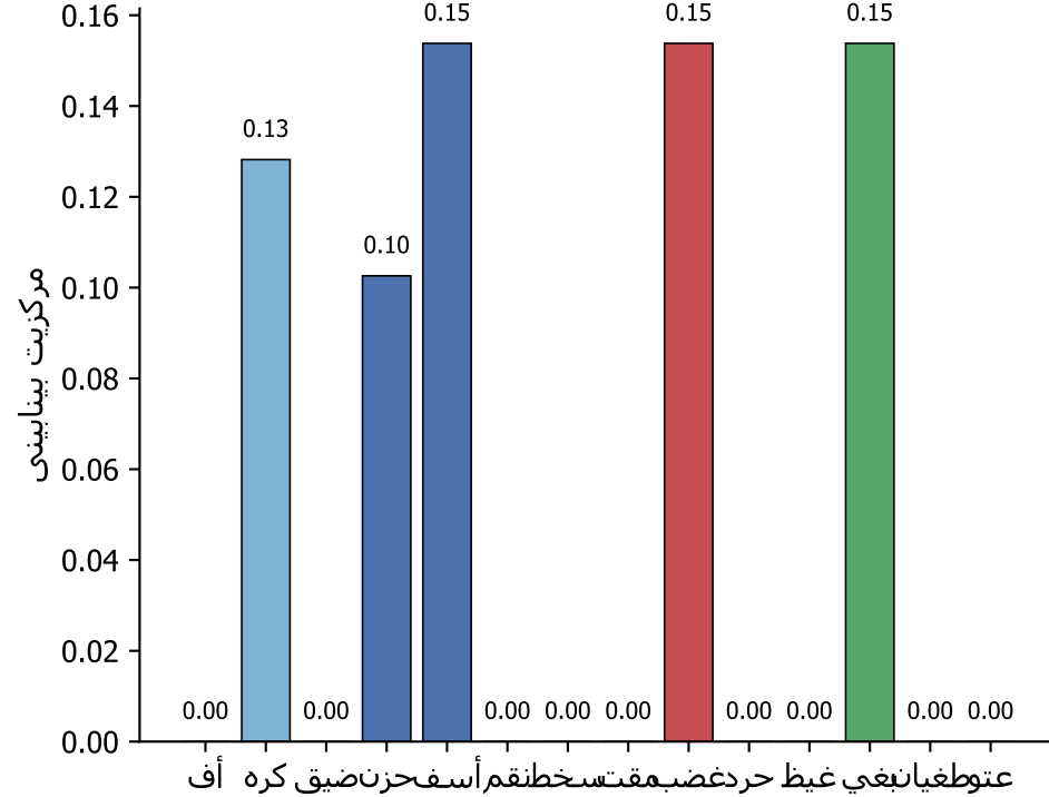
ب) مرکزیت بینابینی
