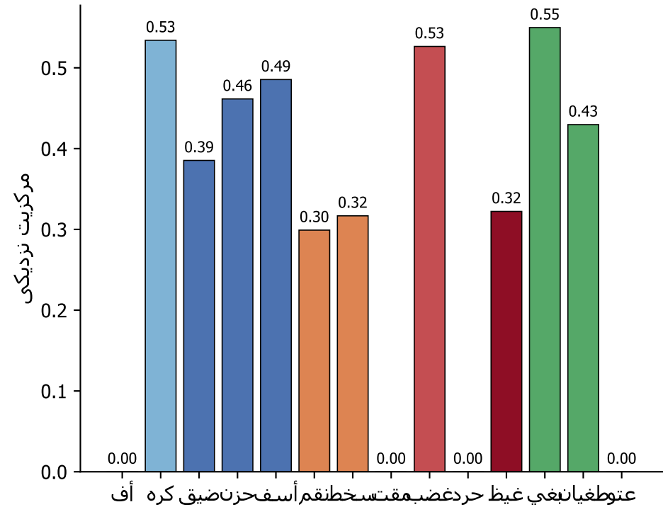
ج) مرکزیت نزدیکی
