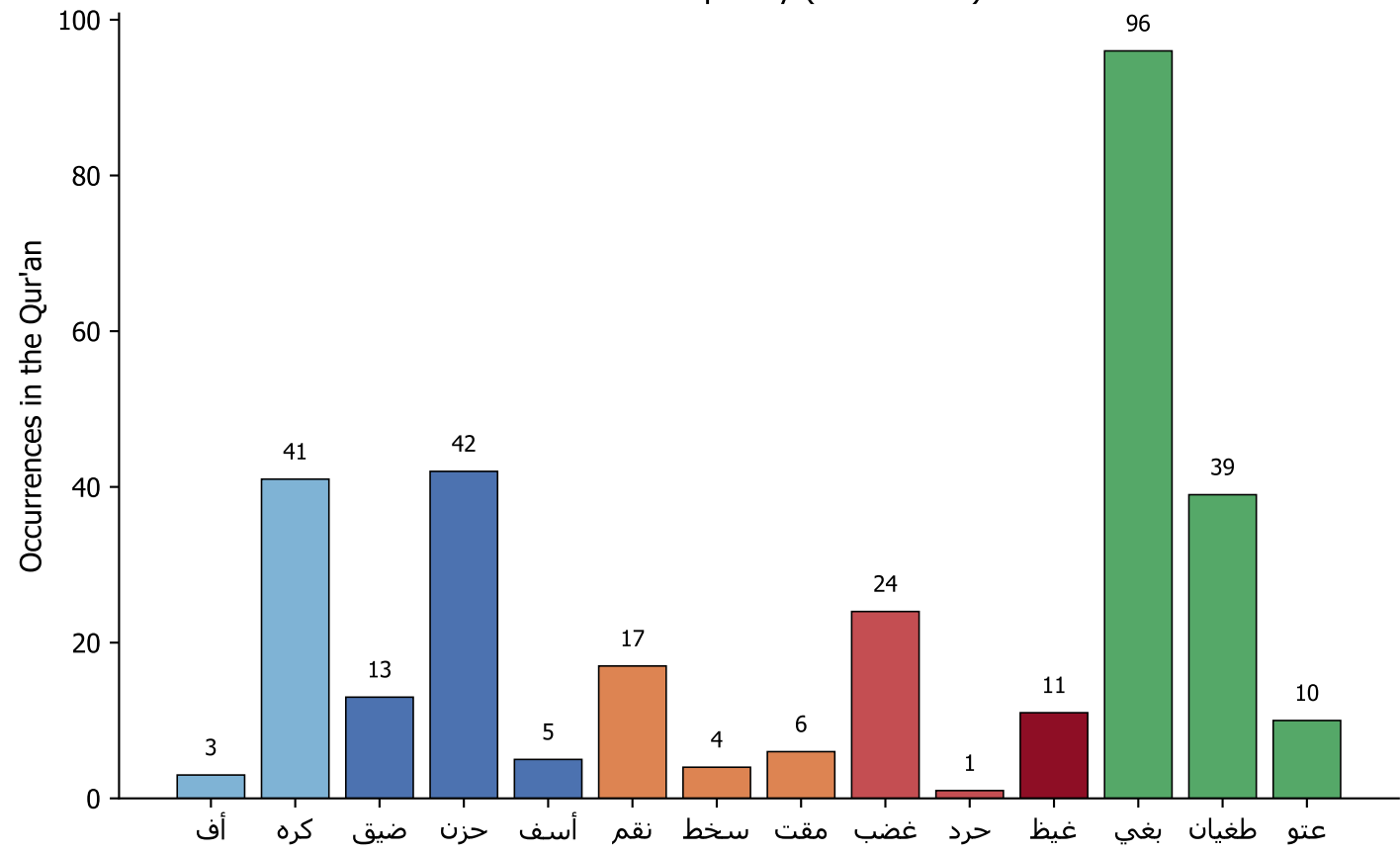
Per-root frequency (linear scale)
