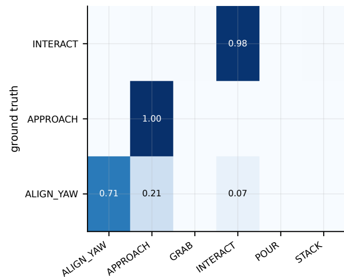
Qwen2.5-3B-Oracle-LoRA
