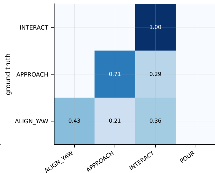
Qwen2.5-3B-Oracle→WoZ-LoRA
