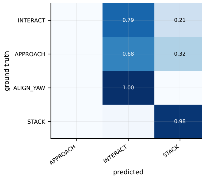
H2 Always-Ask
