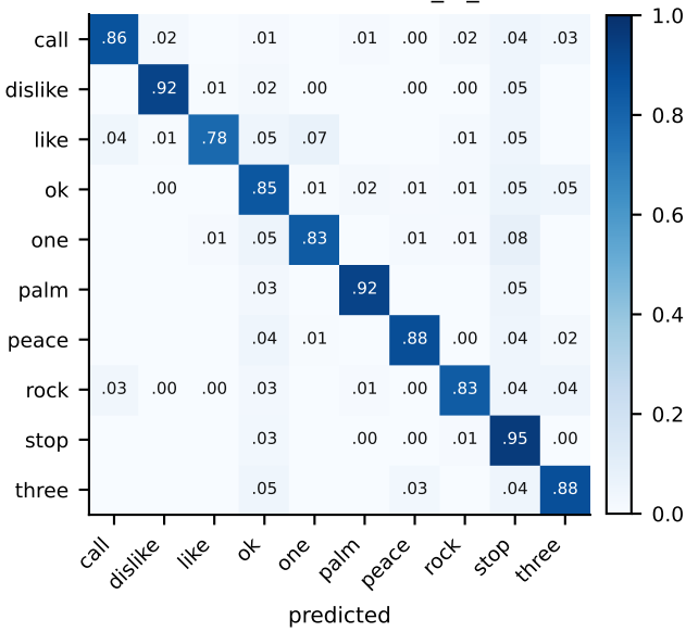
confusion matrix — e1_rs_test
