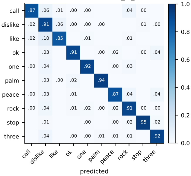
confusion matrix — e1_rs_val
