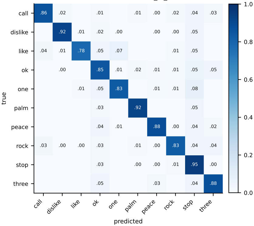
confusion matrix — e1_rs_test
