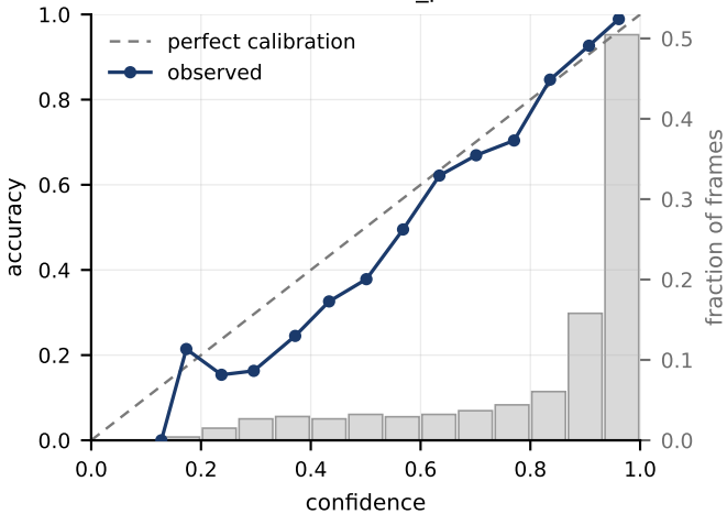
calibration — e1_pseudo
